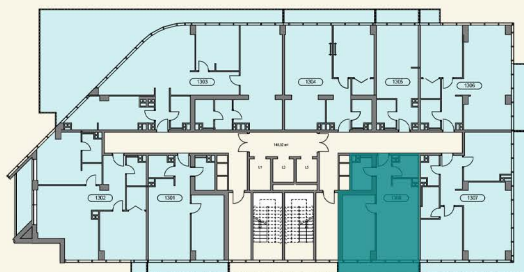
Mərtəbə planı
