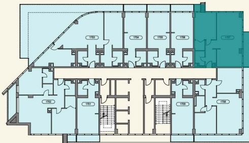
Mərtəbə planı
